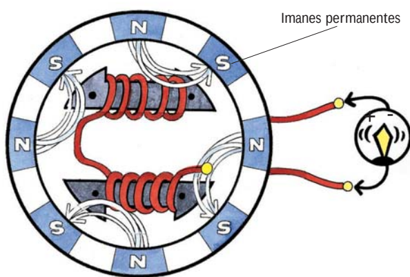
VOLANTE MAGNÉTICO
