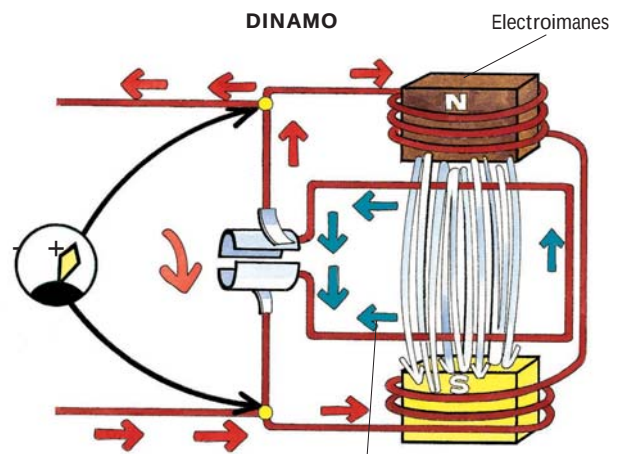
DINAMO
