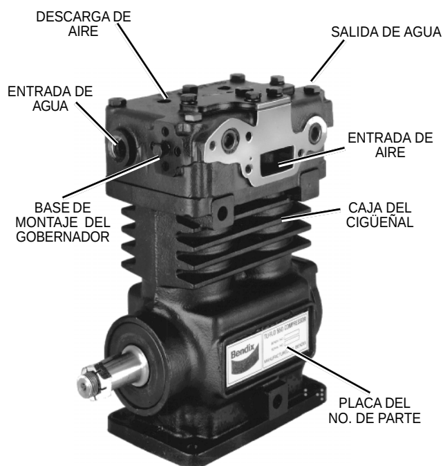
COMPRESOR DE AIRE BENDIX® TU-FLO® 550 (EXTERIOR)
