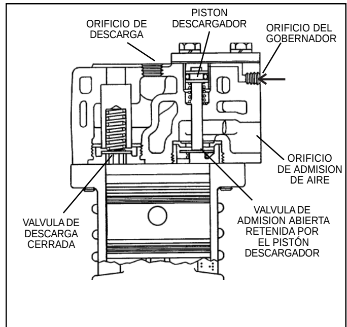
FIGURA 6 - OPERACION DE DESCARGA
