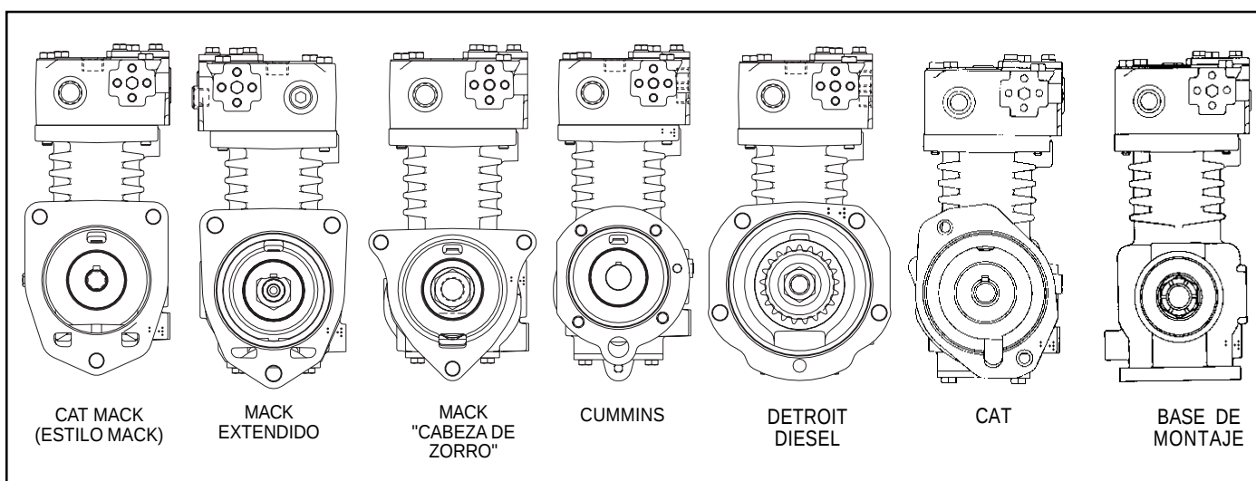
FIGURA 2 - CONFIGURACIONES DEL REBORDE
