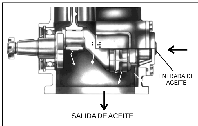
FIGURA 7 - LUBRICACION
