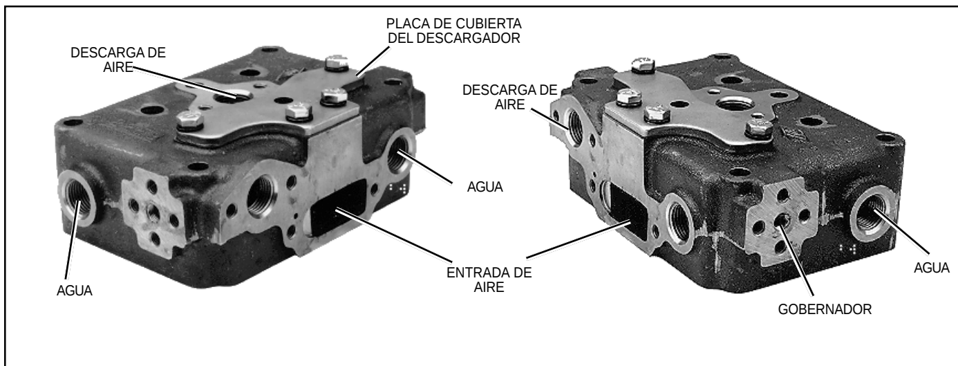
FIGURA 1 - CABEZA DEL CILINDRO
