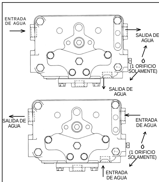
FIGURA 8 - ENFRIAMIENTO INDUCCION DE AIRE
