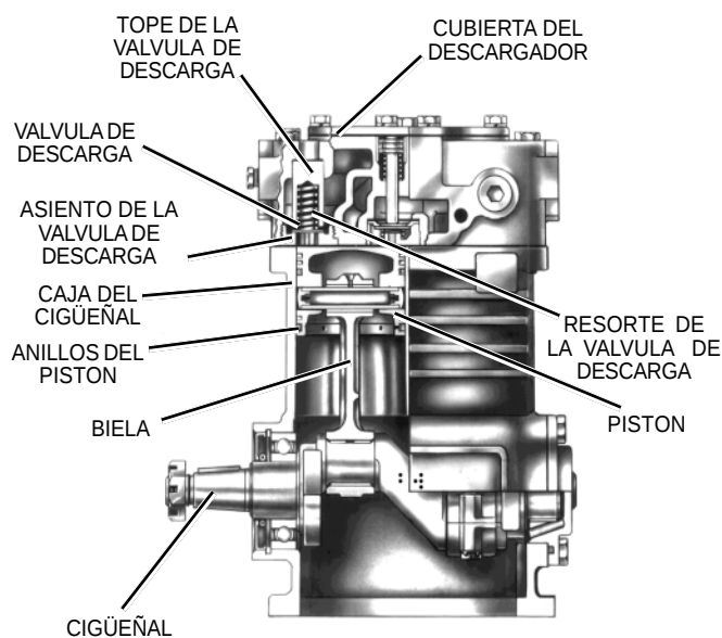
COMPRESOR DE AIRE BENDIX® TU-FLO® 550 (SECCION TRANSVERSAL)
